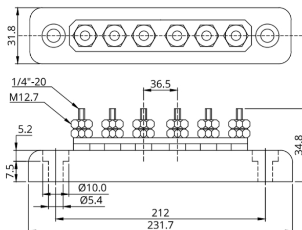
Sběrnice 150 A se 6 svorovými výstupky (kryt není zobrazen)
