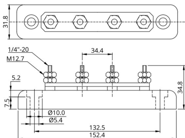
Zbernica 150 A so 4 svorovými svorkami a krytom
