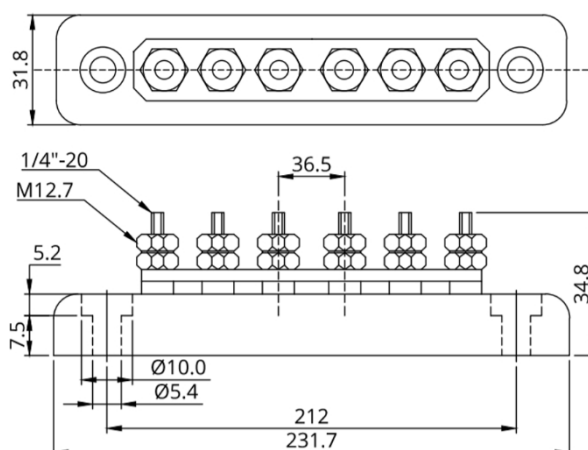
Zbernica 150 A so 6 svorovými vývodmi (kryt nie je zobrazený)
