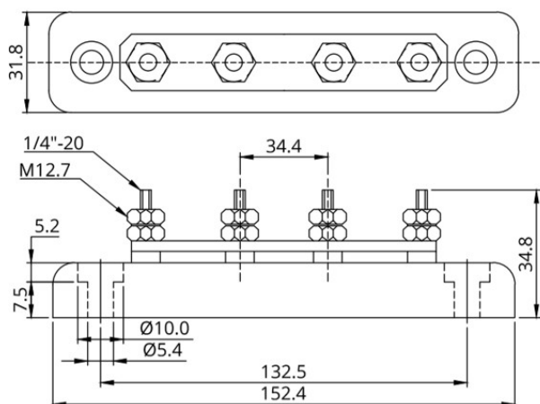
Sběrnice 150 A se 4 svorovými výstupky a krytem
