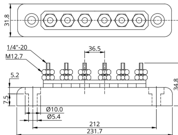
Sběrnice 150 A se 6 svorovými výstupky (kryt není součástí dodávky)
