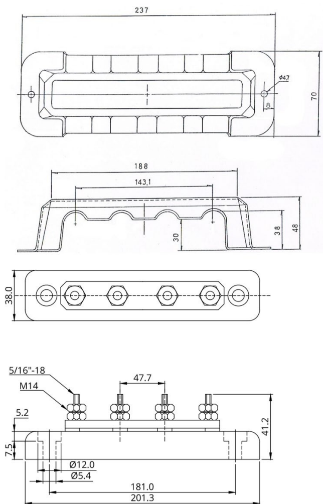
Zbernica 250 A so 4 svorkami a krytom
