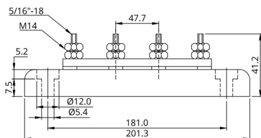
Přípojnice 250 A se 4 šroubovými svorkami a krytem
