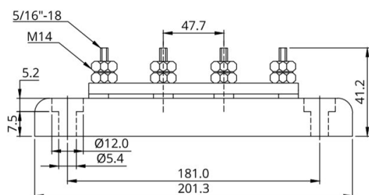
Zbernica 250 A so 4 skrutkovými svorkami a krytom
