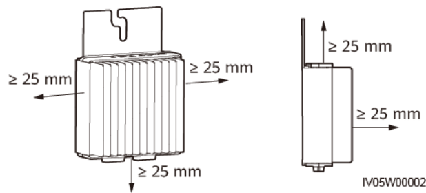
Abbildung 3-1 Abstandsanforderungen
