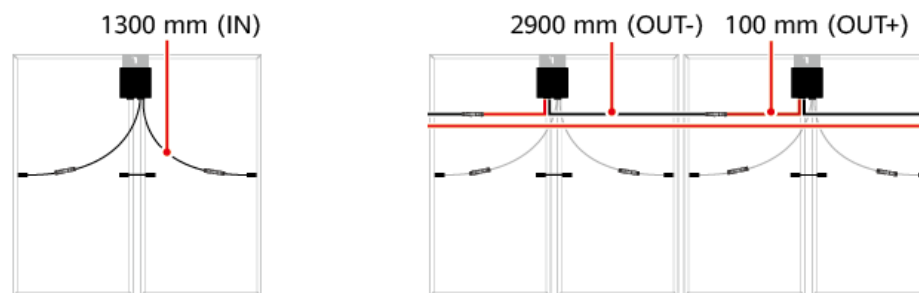
Abbildung 3-3 Optimierer mit langen Eingangsstromkabeln
