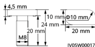
Abbildung 3-6 Schraubenabmessungen
