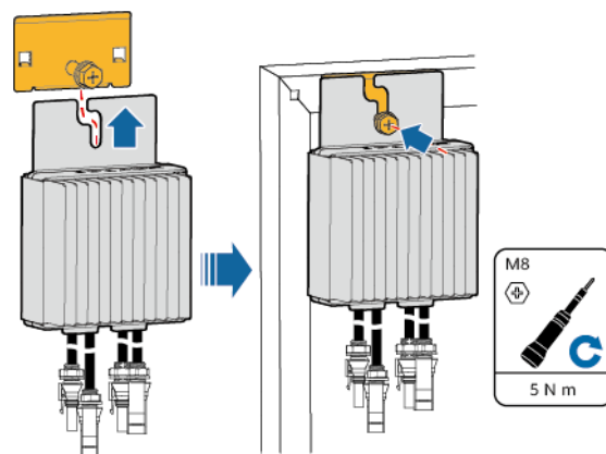
Abbildung 3-8 Installieren des Optimierers mit einer Montagehalterung des Rahmens am PV-Modul-Rahmen (Frontmontage)
