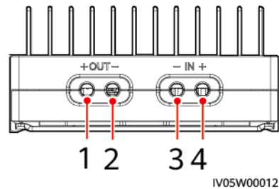
Abbildung 2-3 Ports
