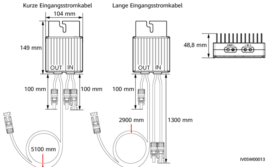
Abbildung 2-4 Abmessungen des Optimierers
