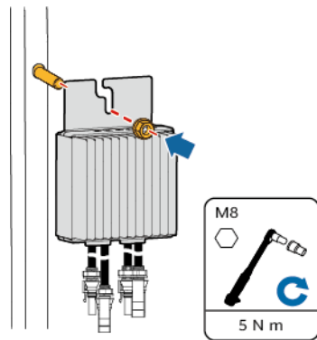
Abbildung 3-7 Installieren des Optimierers mit einer Schraubenbaugruppe am PV-Modul-Rahmen
