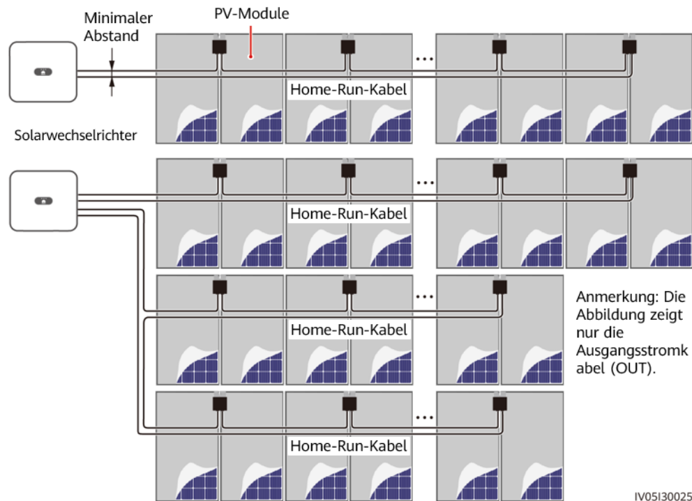
Abbildung 3-12 Erforderliches Kabelverlegung
