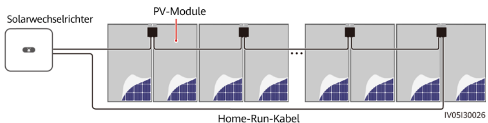
Abbildung 3-13 Verbotenes Kabelverlegung
