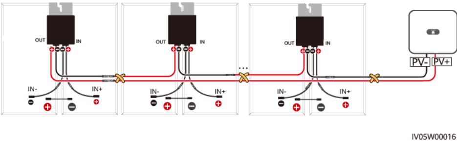
Abbildung 2-1 Anwendungsszenario (Optimierer für alle PV-Module konfiguriert)
