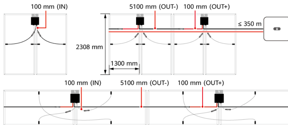
Abbildung 3-2 Optimierer mit kurzen Eingangsstromkabeln
