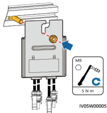
Abbildung 3-5 Installieren des Optimierers mit einer T-förmigen Schraube auf dem Aluminium-Strangpressprofil
