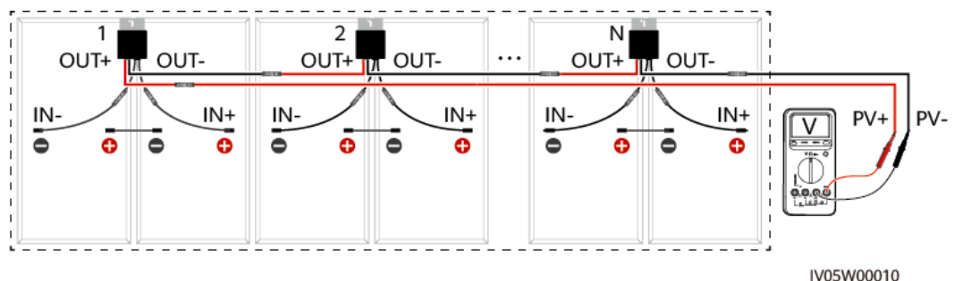
Abbildung 3-11 Messen der PV-String-Spannung
