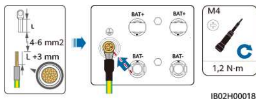
Abbildung 5-3 Anschließen des PE-Kabels
