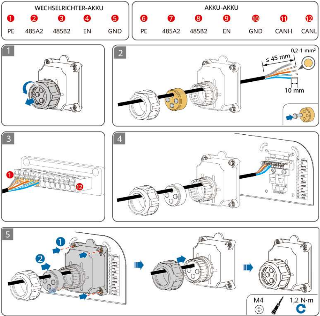
Abbildung 5-6 Signalanschlussverbindungen
