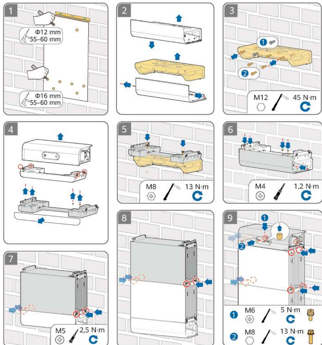
Abbildung 4-6 Wandmontage
