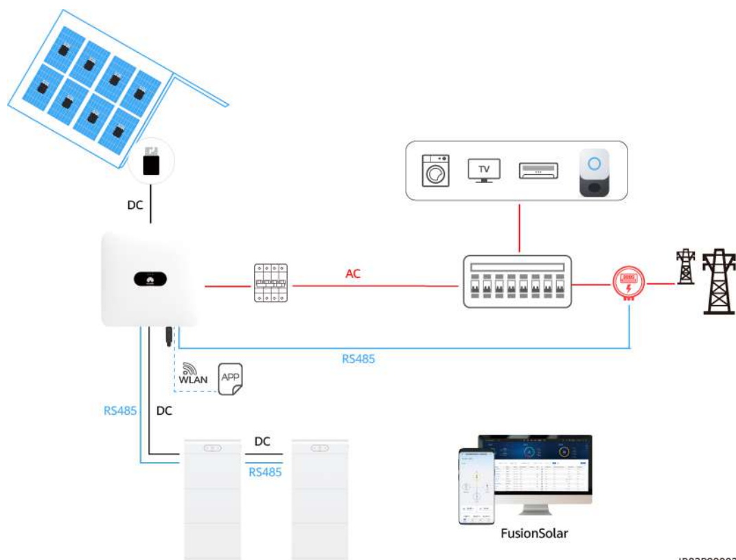
Abbildung 2-7 Netzgekoppeltes Szenario
