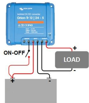
Intrerupator on-off conectat la polul plus al bateriei
