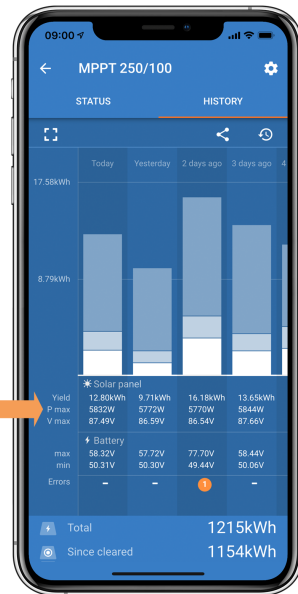
VictronConnect-App mit Historie Pmax-Wert.
