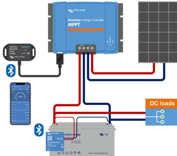
Exemplu de rețea VE.Smart formată dintr-un Smart Battery Sense și un încărcător solar.
