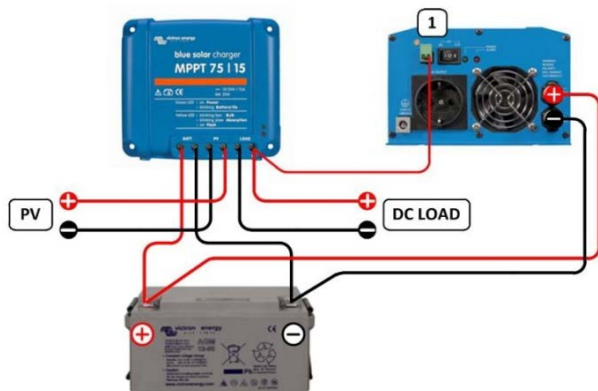
Figura 5: Invertoarele Victron modelele Phoenix 12/800, 24/800, 12/1200 și
