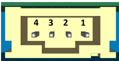
Figura 1b: numerotarea pinilor portului de comunicație VE.Direct, modele de 75 V
