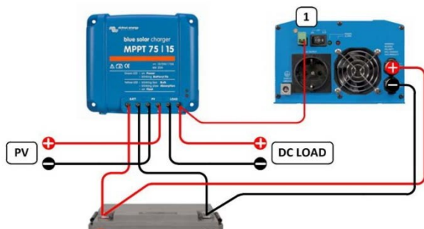
Figura 5: Invertoarele Victron modelele Phoenix 12/800, 24/800, 12/1200 și 24/1200 pot fi controlate prin conectarea conexiunii din partea dreaptă (1) a telecomenzii inverterului direct la ieșirea de sarcină a încărcătorului solar. În mod similar, toate invertoarele Phoenix VE.Direct pot fi controlate prin conectarea la conexiunea din partea stângă a telecomenzii
