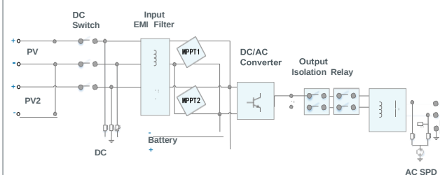
Schema circuitului
