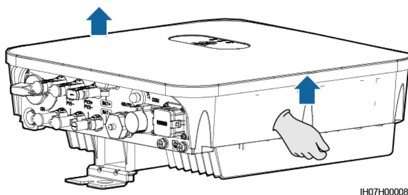
Figura 4-6 Deplasarea unui dispozitiv SUN2000
