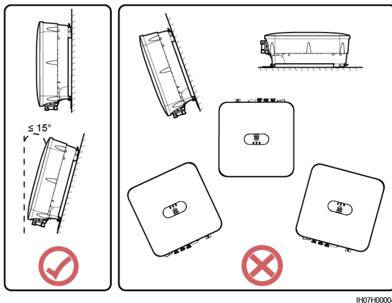
Figura 4-1 Unghiul de instalare
