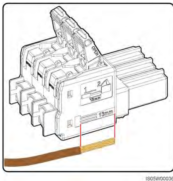
Figura 5-9 Lungimea pentru dezizolarea cablurilor
