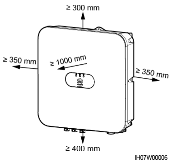
Figura 4-2 Spațiul de instalare
