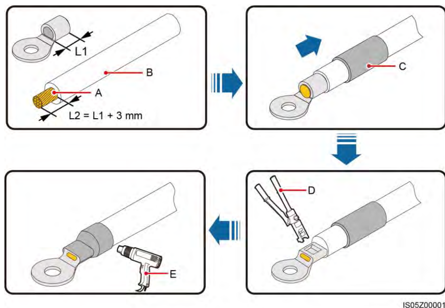
Figura 5-2 Sertizarea unei borne OT
