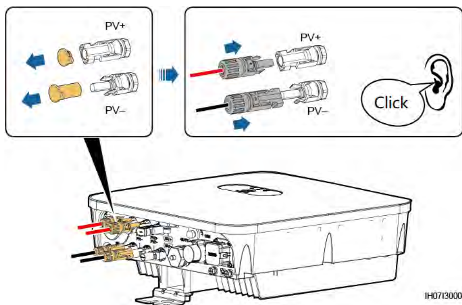
Figura 5-15 Conectarea cablurilor electrice de intrare c.c.
