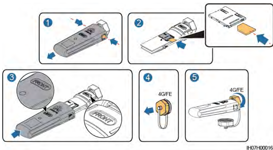
Figura 5-4 Instalarea unui 4G Smart Dongle
