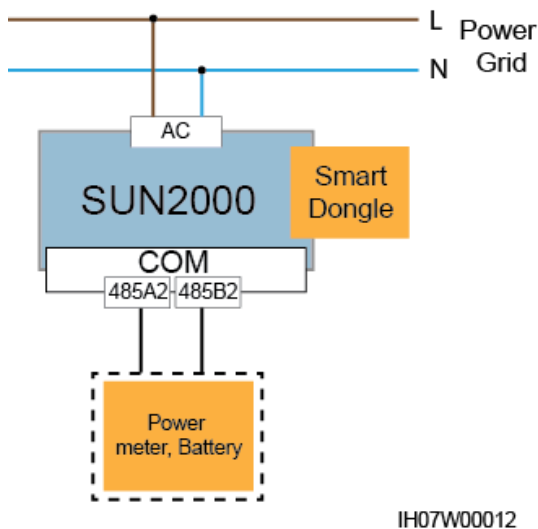
Figura 5-19 Un singur dispozitiv SUN2000
