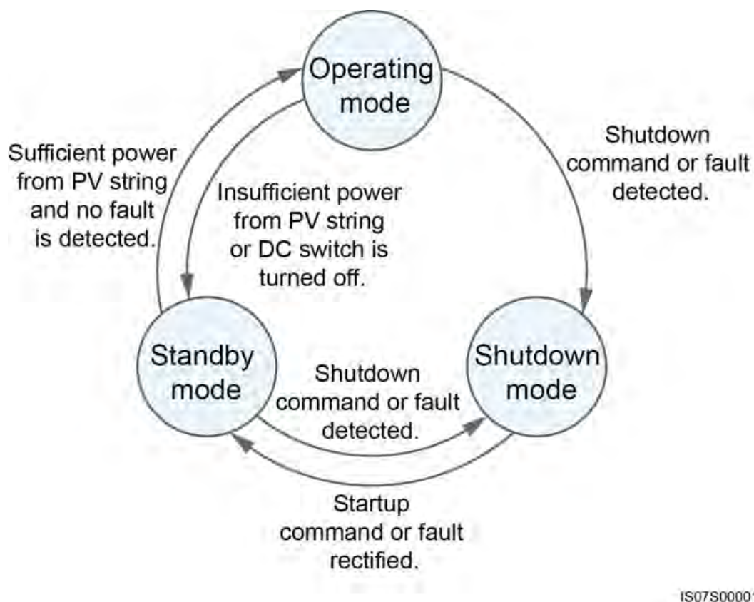
Figura 2-8 Modurile de funcționare
