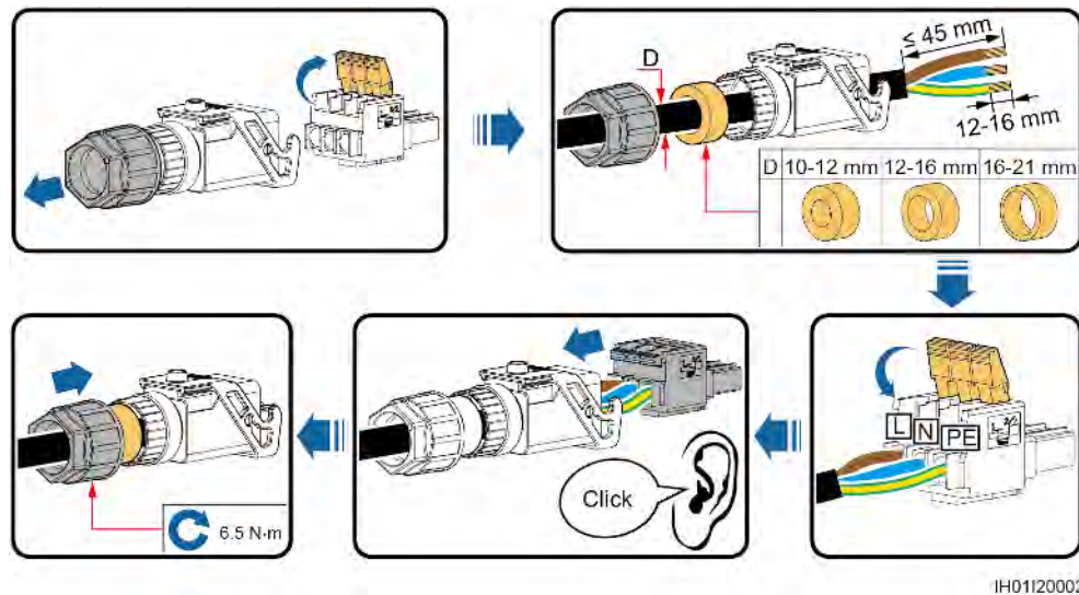
Figura 5-7 Asamblarea unui conector c.a. (fir cu trei conductoare)
