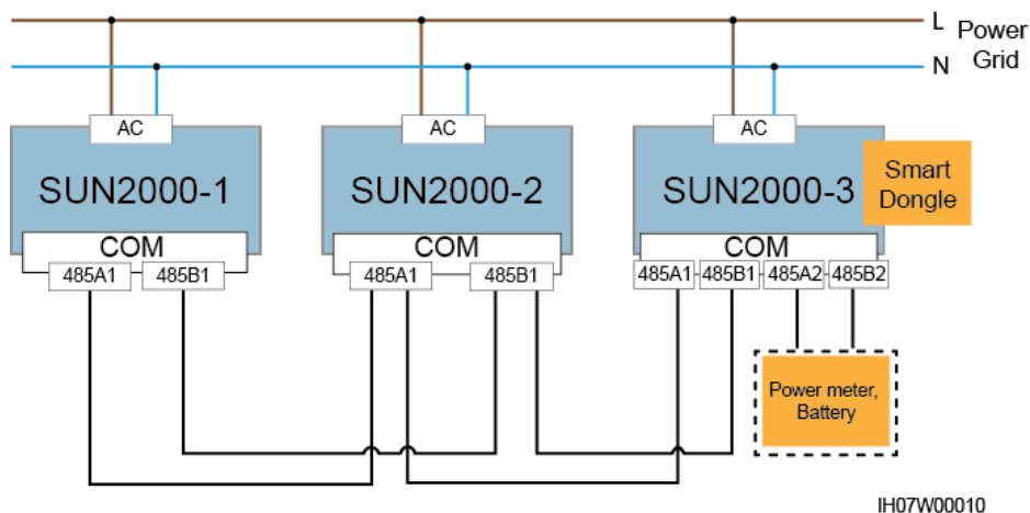
Figura 5-21 Conexiune rețea în fază
