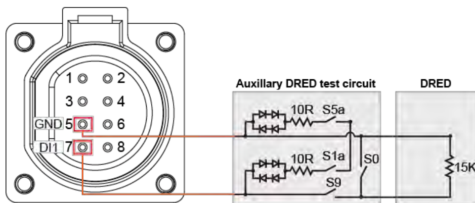
Figura 7-19 Diagrama de cablare pentru funcția DRM
