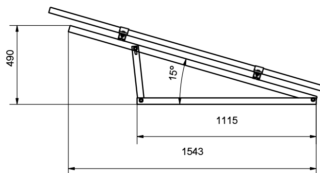
FIG. 1 Dimensiunile modelului 07-S-15N
