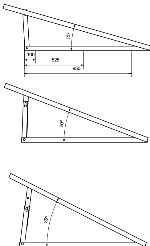
Fig. 1K-07-M-RN: dimensiunile structurii în funcție de unghiul utilizat
