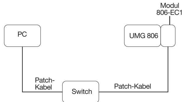
Abb. Anschlussbeispiel: UMG 806 mit Modul 806-EC1 und PC benötigen eine feste IP-Adresse (Parameter 205 = 0).
