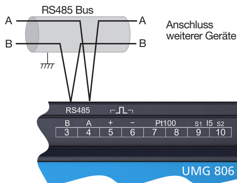
Abb.-Bsp.: RS485-Schnittstelle des UMG 806 (inmitten einer Bus-Topologie)
