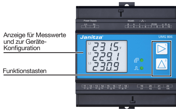
Abb. Messwert-Anzeige UMG 806 "Spannung L1-N, L2-N und L3-N" und Funktionstasten.
