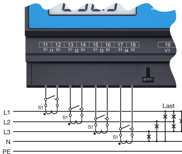
Abb. Anschlussbeispiel „Strommessung“ beim UMG 806.
