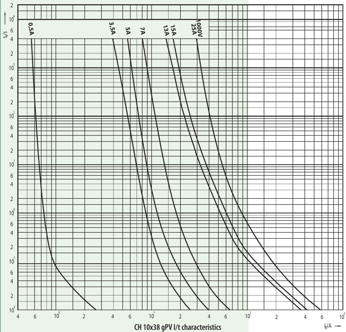
Caratteristiche I/t CH 10x38 gPV
