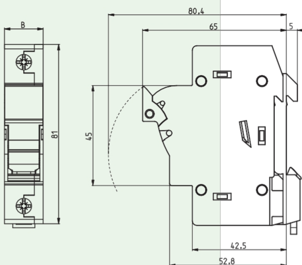
Ausführung mit Adapter
