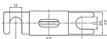
Držiak poistky pre ANL poistku
