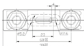
Držiak poistky pre ANL poistku
