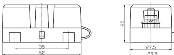
Držiak poistky pre poistky MIDI
