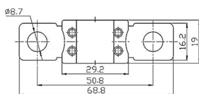
MEGA poistka
