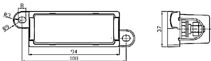
Držiak poistky pre poistku MEGA
