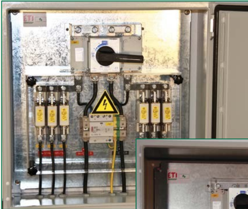
DC-Anschlusskasten (NH-gPV-Sicherungen)
