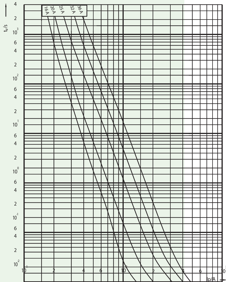
Kapitel 14 PV-I/t-Kennlinien
