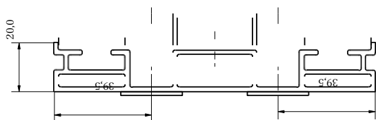
Fig. 3 Șină din aluminiu K-66-1
