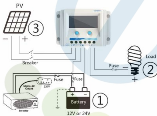
Obr 3 Diagram pripojenia
