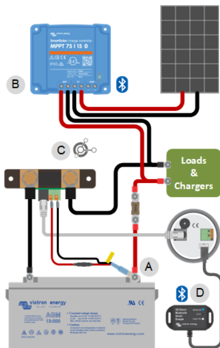
Exemplu de sistem care conține un sistem de monitorizare a bateriei cu senzor de temperatură și un încărcător solar, ambele utilizând rețeaua VE.Smart.
