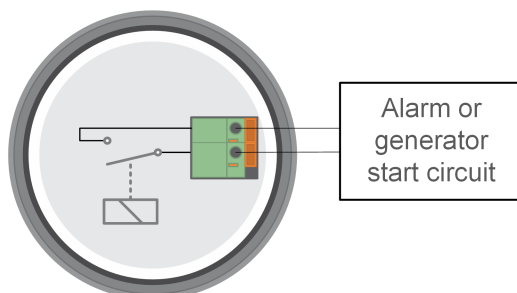
Diagrama de cablare internă a sistemului de monitorizare a bateriei cu releul într-o stare fără alimentare conectat la o alarmă externă sau la un circuit de pornire a unui generator.
