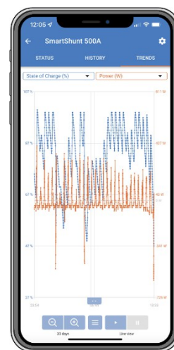
Uložené trendy pre SmartShunt
