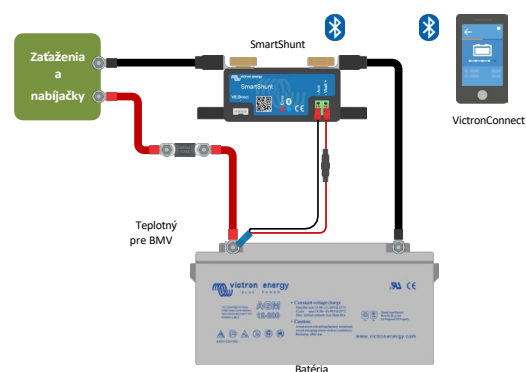
Meranie teploty batérie
