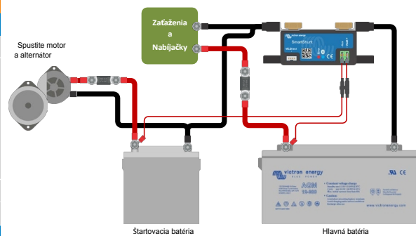
Meranie napätia štartovacej batérie
