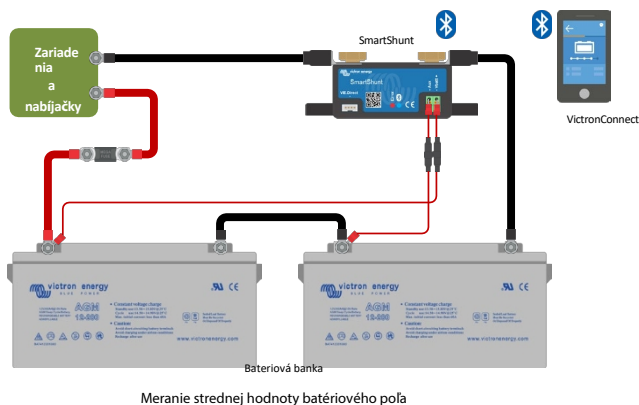
Meranie strednej hodnoty batériového poľa
