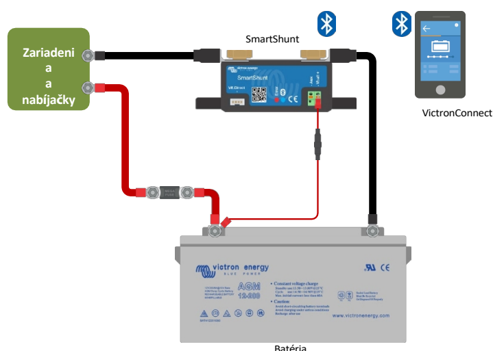
Základné zapojenie SmartShunt
