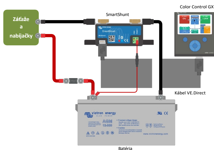
Pripojenie zariadenia SmartShunt k zariadeniu GX
