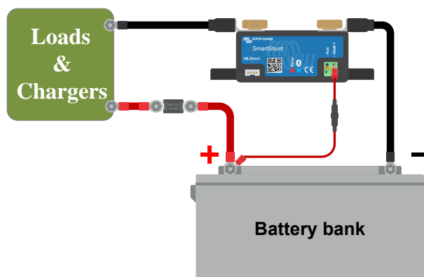
Instalarea sistemului de monitorizare a bateriei de bază.
