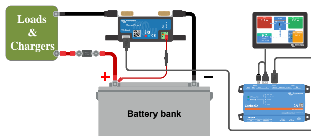
Sistemul de monitorizare a bateriei este conectat la un Cerbo GX și la un ecran GX Touch.
