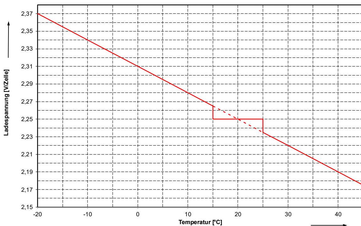
Abbildung 7.2.1-1 - Temperaturabhängige Anpassung der Ladeerhaltungsspannung für Batterietypen mit einer Ladeerhaltungsspannung von 2,25 V/Zelle bei T_{nenn}
