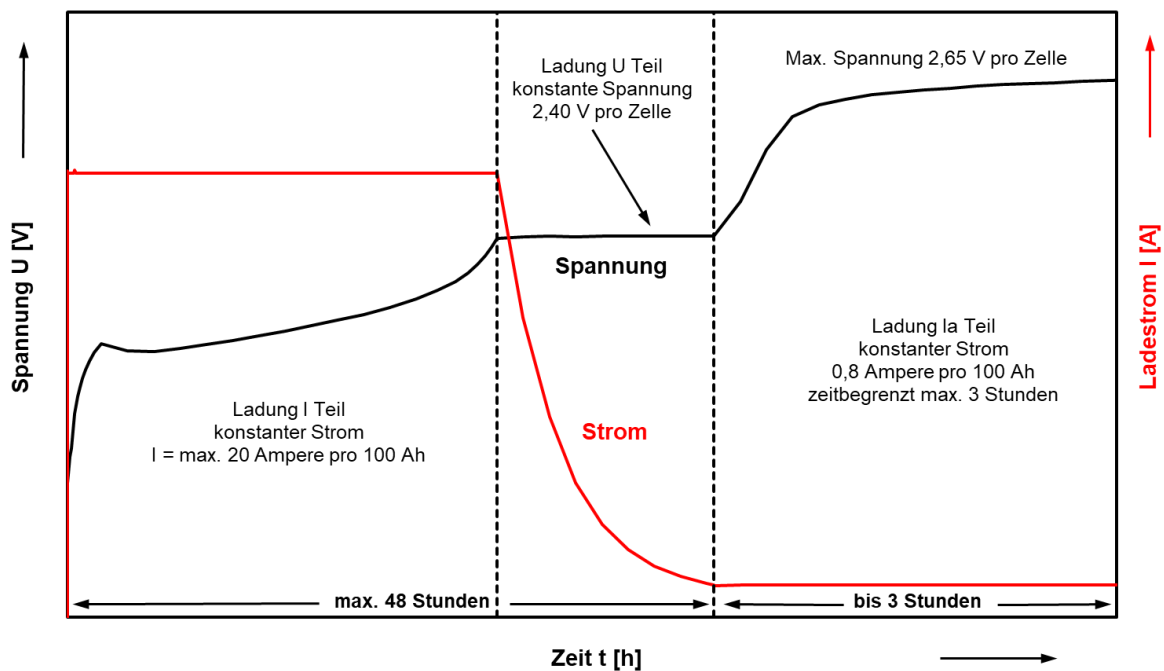
Abbildung 8-2 - Kennlinie IU Ia
