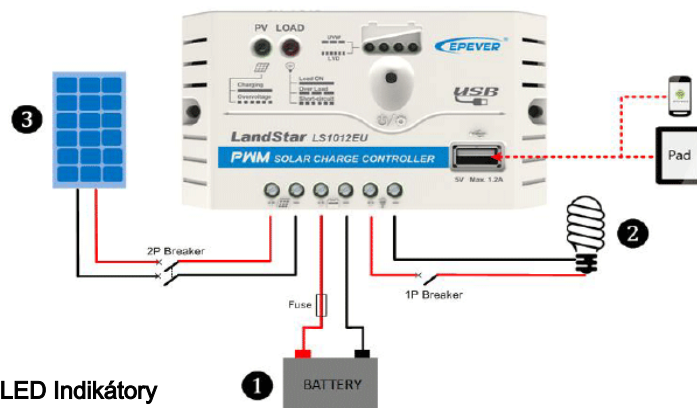
Obrázok 2 - diagram zapojenia
