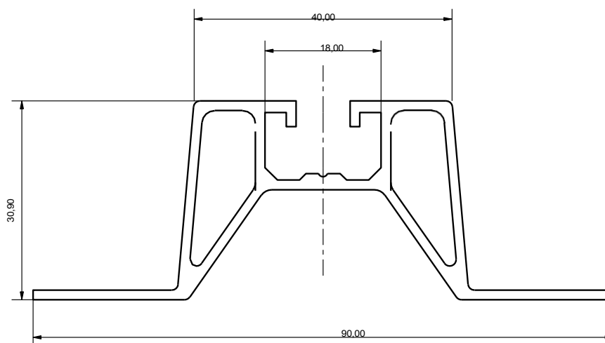
Fig. 2 Dimensiunile elementului K-14-N
