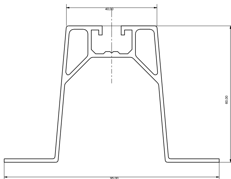
Fig. 1 Dimensiunile elementului K-14
