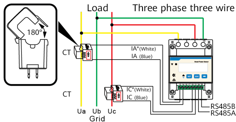
Abbildung 4-3 Drehstrom-Dreileiter (unterstütztes Modell: DTSU666-H 250 A/50 mA)
