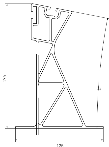
Obr. 1 Hliníkový montážny držiak K-45-7, vysoký
