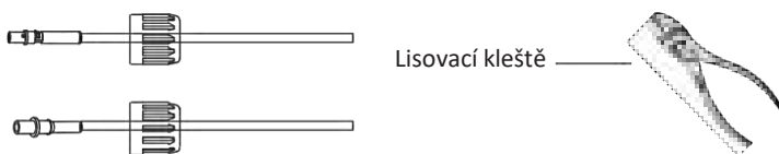
Obr. 3.4 Lisování kontaktního kolíku na vodič
