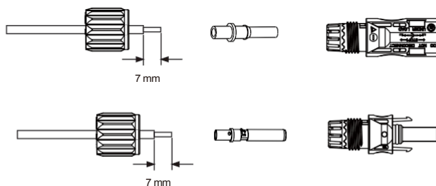
Fig. 3.3 Demontați piulița capacului conectorului
