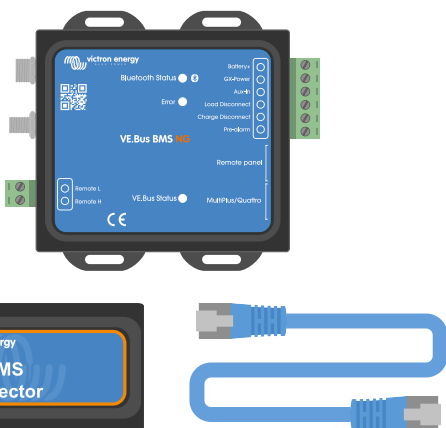
VE.Bus BMS NG, detector de rețea VE.Bus BMS și cablu RJ45 UTP
