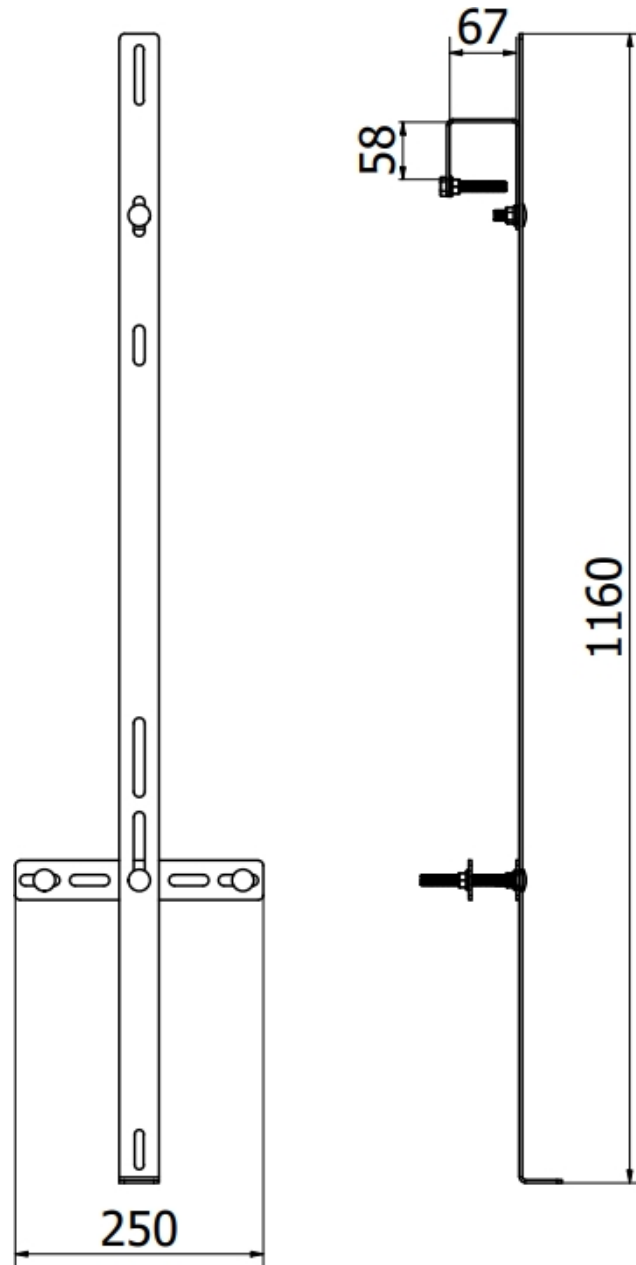
Abb. 1 Abmessungen der Konstruktion
