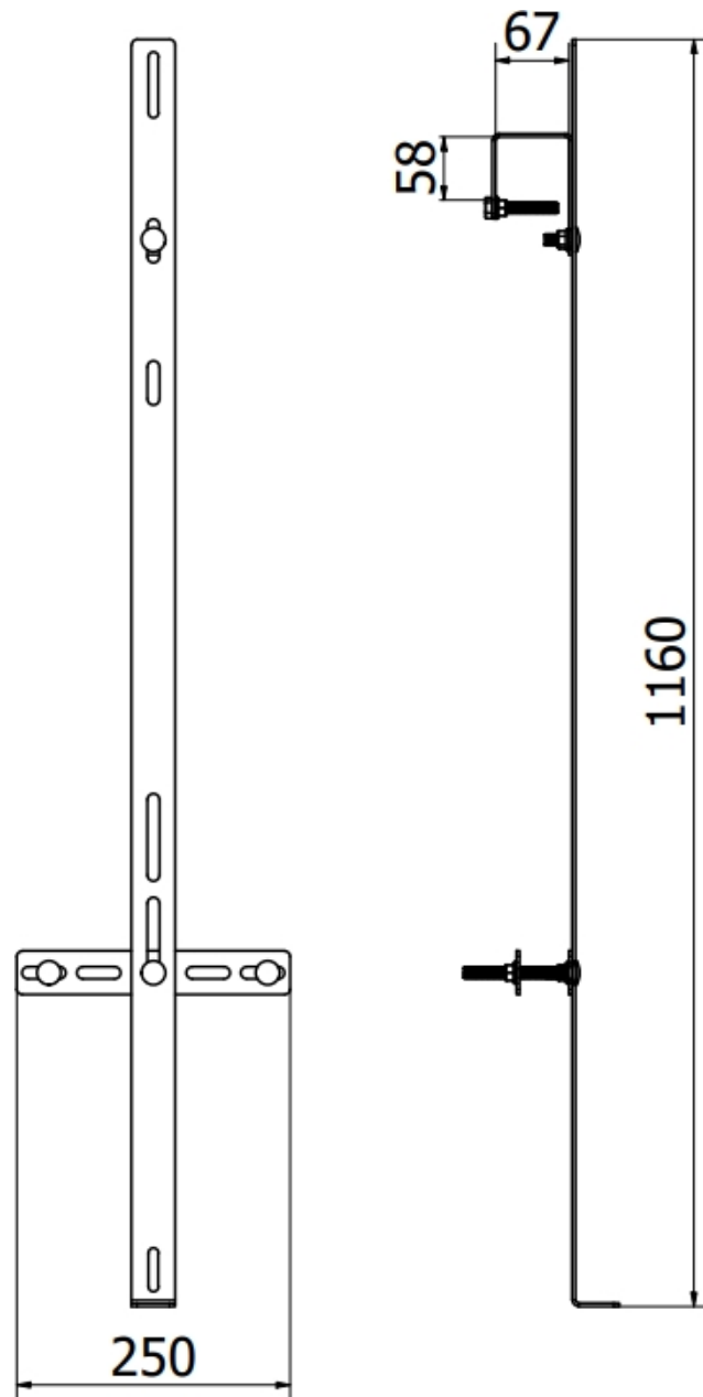
Fig. 1 Dimensiunile structurii
