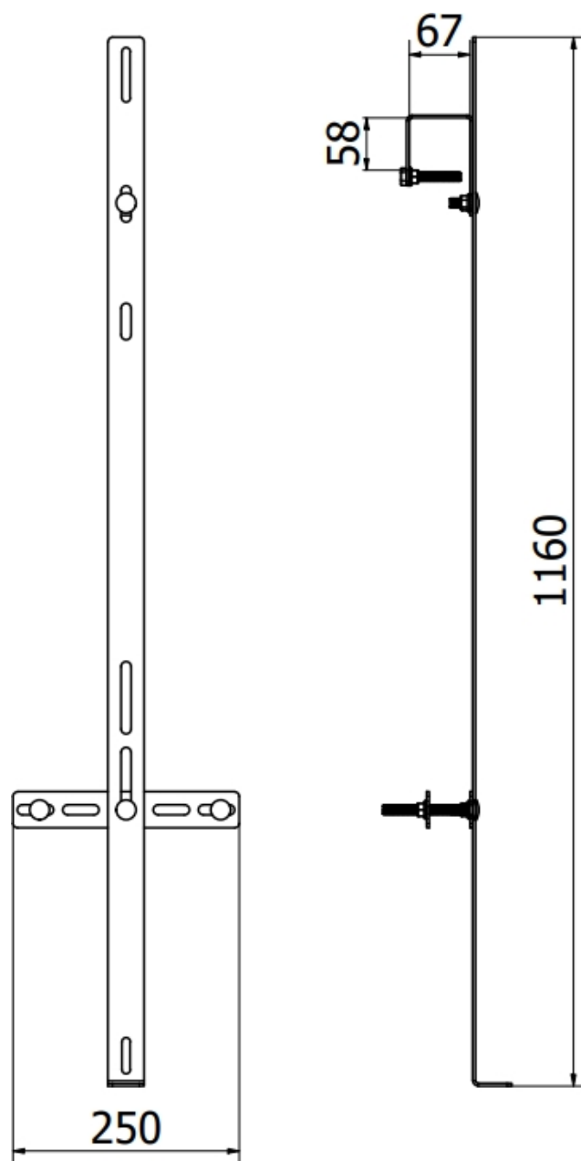
Obr. 1 Rozměry konstrukce
