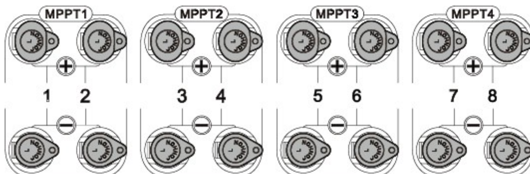
Obrázek 5-11 Svorky pro vstup stejnosměrného proudu
