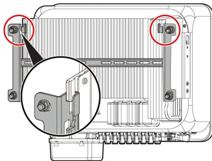
Obrázek 4-13 Instalace střídače
