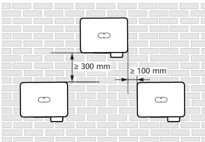
Obrázek 4-5 Dvouvrstvá instalace do trojúhelníku (doporučeno)
