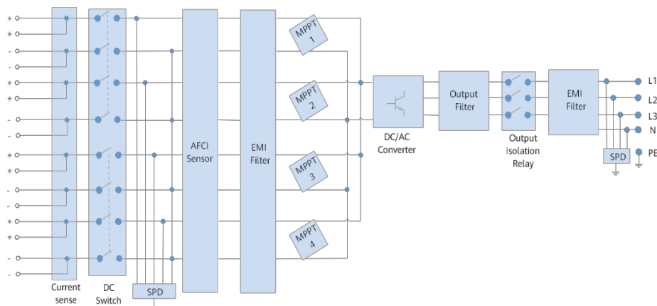
Obrázek 2-7 Schématický diagram
