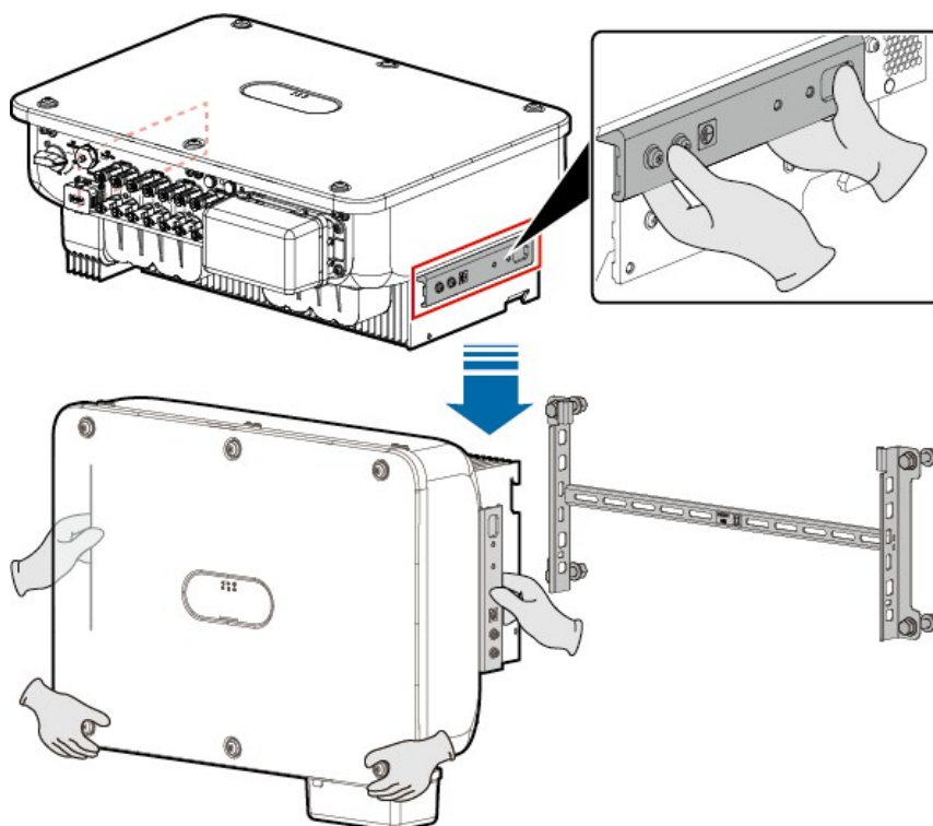
Obrázek 4-10 Přemísťování střídače
