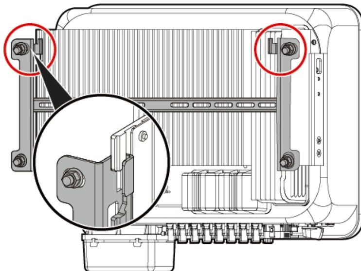
Obrázek 4-16 Instalace střídače
