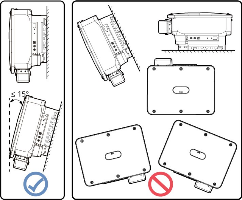
Obrázek 4-9 Úhel instalace
