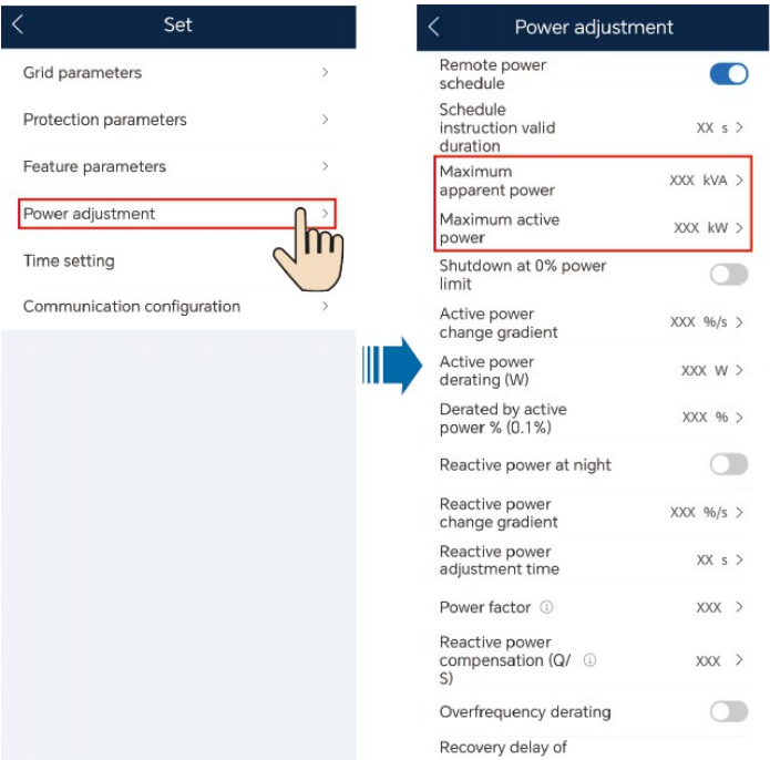
Obrázek 7-9 Řízení zdánlivého výkonu
