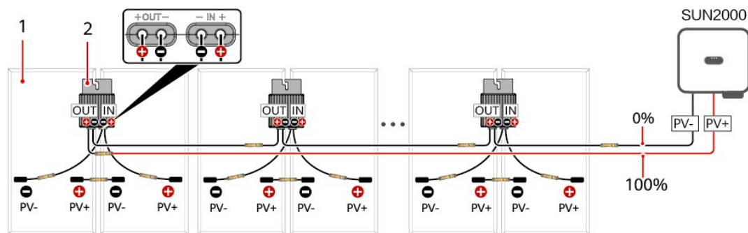
Obrázek 8-2 Definice procenta polohy zkratu (při nakonfigurovaných optimalizátorech)
