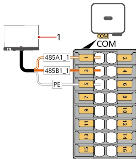
Obrázek 5-32 Zapojení kabelů
