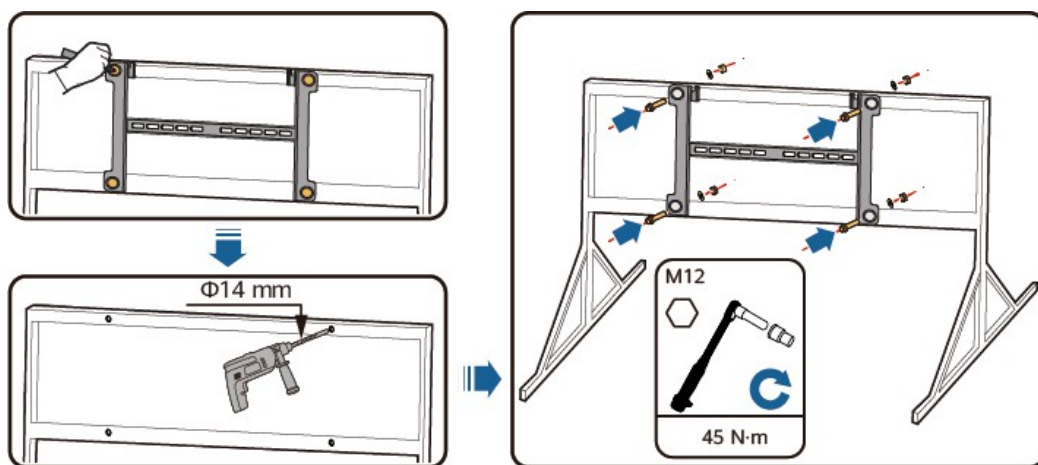
Obrázek 4-15 Upevnění montážního držáku
