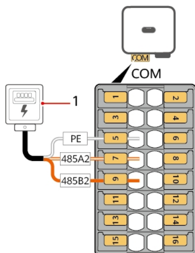
Obrázek 5-35 Zapojení kabelů
