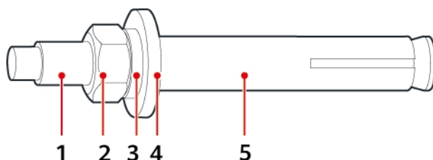
Obrázek 4-11 Konstrukce rozpínacího šroubu
