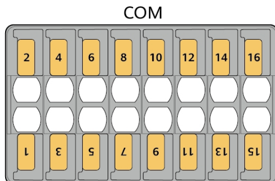
Obrázek 5-26 Definice pinů
