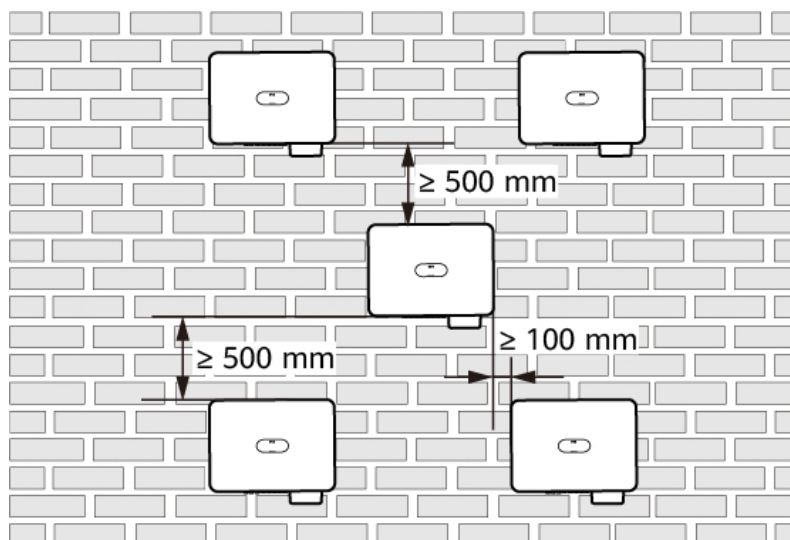
Obrázek 4-6 Třívrstvá trojúhelníková instalace (nedoporučeno)
