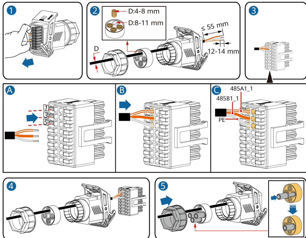
Obrázek 5-33 Instalace kabelu
