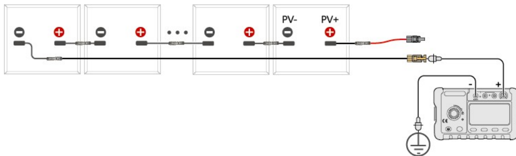
Obrázek 5-16 Měření izolačního odporu fotovoltaického kabelu u každého fotovoltaického řetězce
