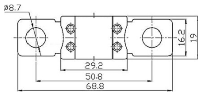
MEGA-Sicherung
