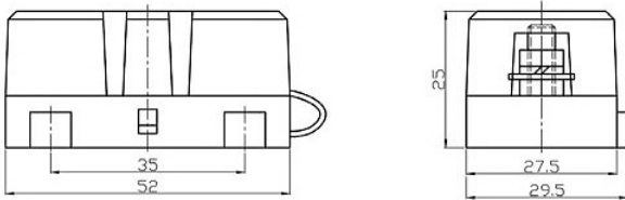
Sicherungshalter für MIDI-Sicherung
