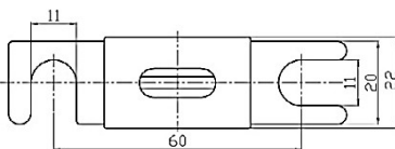
ANL-Sicherung
