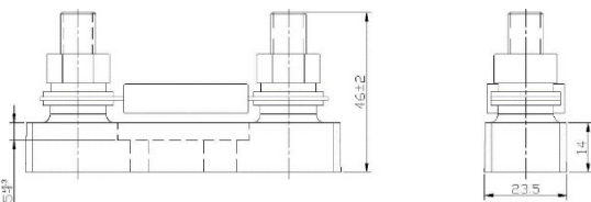
MEGA-Sicherung
